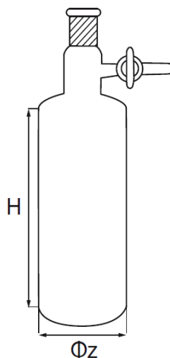
Rys. rysunek poglądowy dotyczący naczynia reakcyjnego/przechowującego Schlenka.
